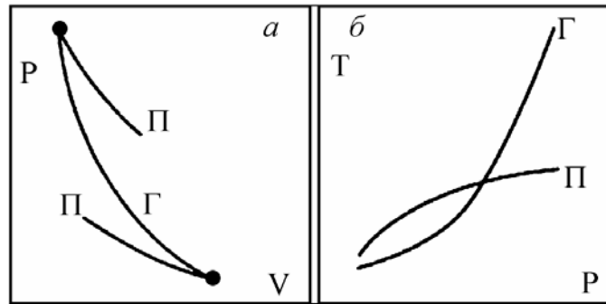
Рис. 4. Адиабаты Пуассона (Π) и Гюгонио (Γ) в координатах: pV - а и pT - б.
