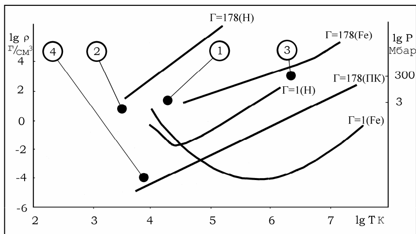
Рис. 3. Фазовая диаграмма «плотность-температура» для водорода и железа (по данным Van Horn, 1991). 1 - состояние вещества внутреннего ядра; 2 - параметры железа, полученные (Boehler, 1993) в экспериментах по ударному сжатию; 3 - \rho T центральной части Солнца; 4 - лабораторный результат (Thomas et al., 1994).
