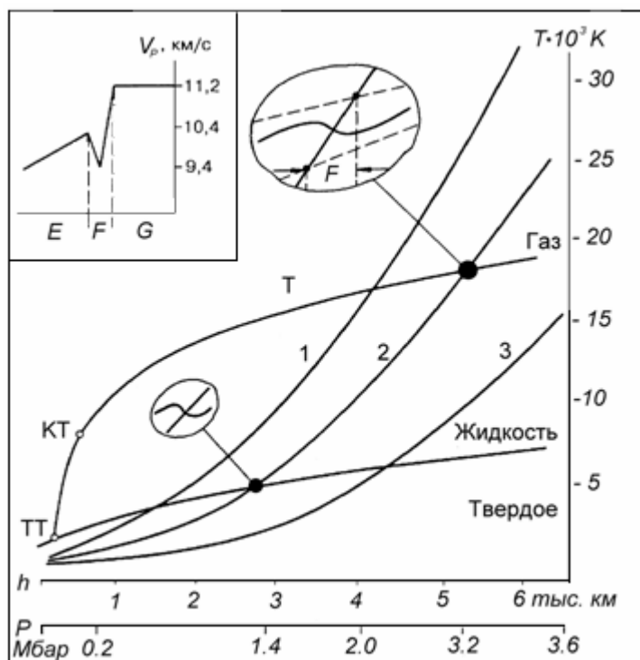
Рис. 5. Диаграмма фазового равновесия вещества Земли (ТТ - тройная точка, КТ - критическая точка, T_p - линия разделяющая фазы при T > T_c и p > p_c ). Адиабаты (А) Гюгонио: 1- рассчитана по формуле (Зельдович, Райзер, 1966), 3- рассчитана по формуле (Brown, McQueen, 1986), 2 - подобрана таким образом, чтобы она пересекалась с диаграммой равновесия на границе ядро-мантия и на границе внутреннего ядра с внешним. В верхнем левом углу - скорости Р-волн в области F-слоя (в интерпретации Джеффриса) - вверху.
