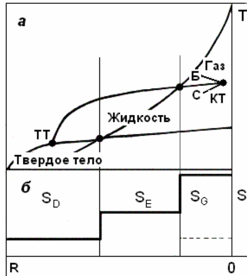
Рис. 2. Распределение температуры (а) и энтропии (б) по оболочкам Земли. а: диаграмма состояния вещества Земли и распределение температуры по адиабате Гюгоню, ТТ – тройная точка, КТ – критическая точка, Б – бинодаль, С – спинодаль.
