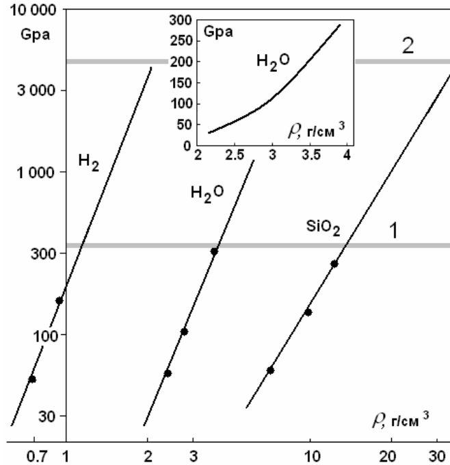
Рис. 1. Зависимость «плотность – давление» для водорода, воды (Cavazzoni, et al., 1999) и окиси кремния.
