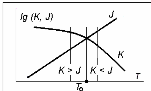
Рис. 6. Изменение \lg скоростей конденсации ( K ) и испарения ( J ) в зависимости от температуры T – вверх.
