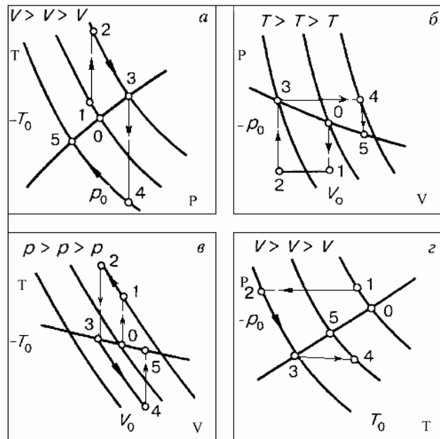
Рис. 7. Термодинамические циклы в области F-слоя -а, -б, -в и в области D''-слоя - г.
