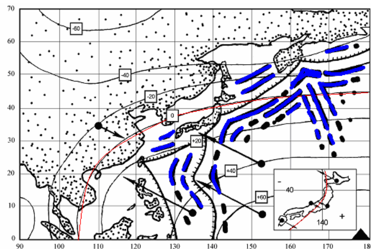
Рис. 2. Карта высот геоида, гравитационных аномалий, направлений и величин дрейфа материков и плит [25, 28, 30]. Черный треугольник внизу справа соответствует максимальному значению высоты геоида. Во вставке (правый нижний угол рисунка) показаны направления скоростей дрейфа литосферы, измеренные в Японии с помощью GPS-системы [31]. Штриховая линия, это линия геодинамического равновесия (аттрактор). При достижении равновесия встречные скорости дрейфа равны нулю.
