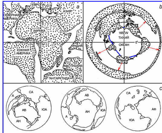
Рис. 4. Предполагаемое первоначальное расположение материков (а); экваториальная проекция периметра Тихого океана и направления дрейфа материков (б) [37]. Расположение материков на сфере радиусом, равным радиусу внешнего ядра Земли (с) [38].
