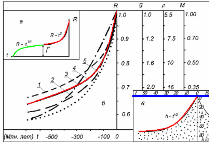
Рис. 5. Изменение земного радиуса R : а) - в течение всего периода эволюции; б) – в течение последних 500 млн. лет эволюции (по данным Кери – 1, Хильденберга – 2, Оуэна – 3, нашей модели – 4) [1]; g - сила тяжести, \rho - средняя плотность Земли 5 – увеличение массы океанов M ; в) – изменение глубины астеносферы h в зоне СОХ, в зависимости от её возраста t .
